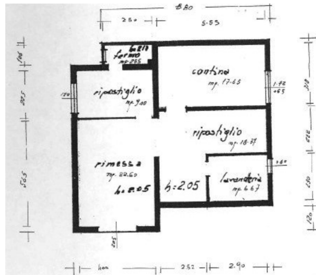
particolare estratto planimetrico abitazione - piano terra e primo
